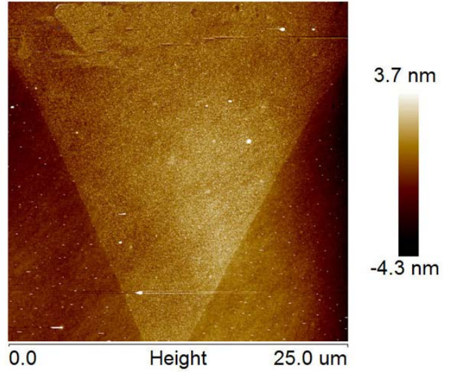
MoS 2 AFM图
